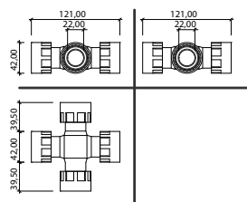
CROSS FxFxFxF 1"
